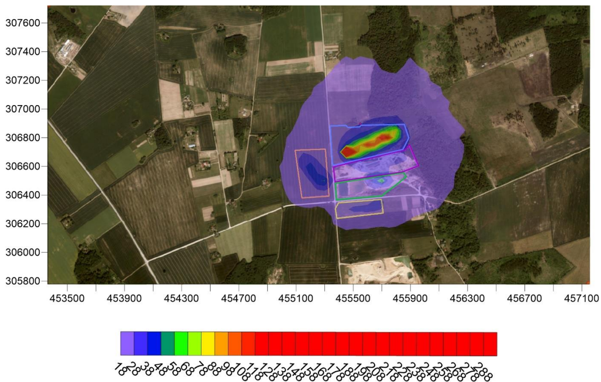
3.10.att. Daļiņu \text{PM}_{10} diennakts 36.augstākās koncentrācijas novērtējums (summārā). 1.alternatīva.
