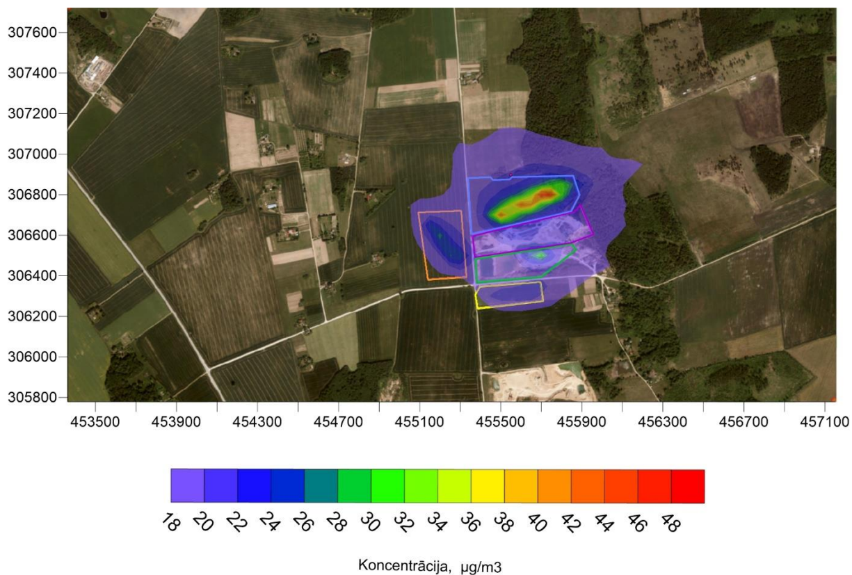
3.7.att. Daļiņu PM 10 gada vidējo koncentrāciju novērtējums (summārā). 1.alternatīva.
