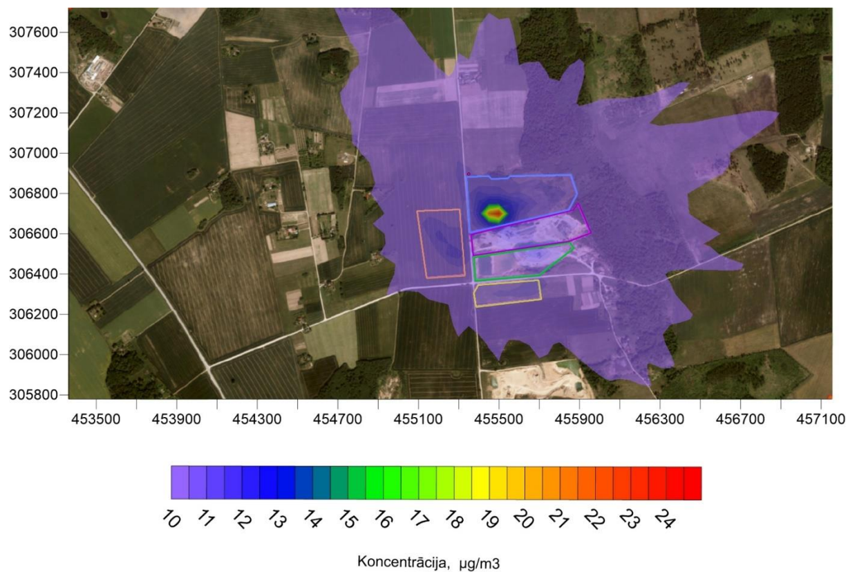
3.13.att. Dalīņu PM 2,5 gada vidējo koncentrāciju novērtējums. 1.alternatīva.
