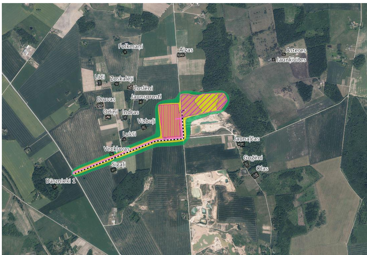
3.18. att. Paredzētās darbības radītā trokšņa rādītāja Ldiena vērtības. 1. transportēšanas alternatīva
