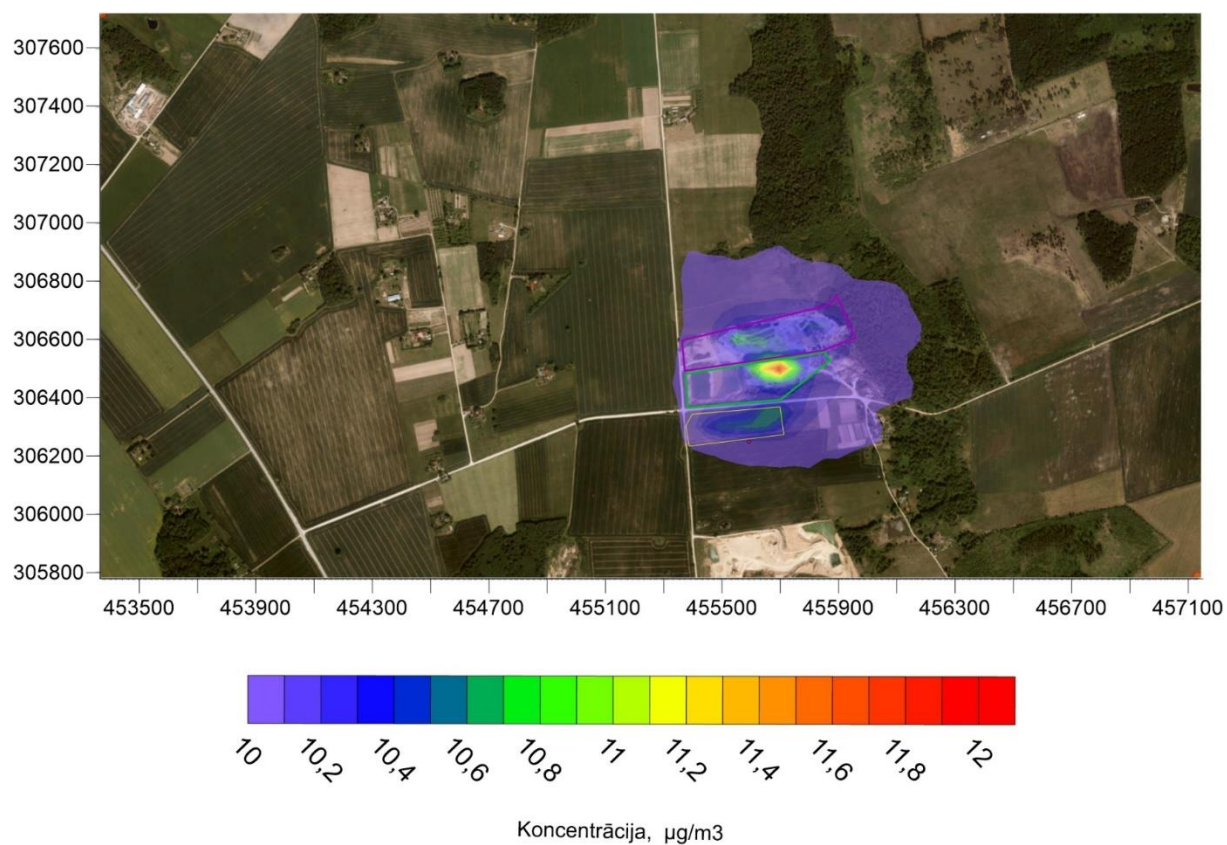
3.12.att. Dalīņu PM 2,5 gada vidējo koncentrāciju novērtējums. Esošā situācija.
