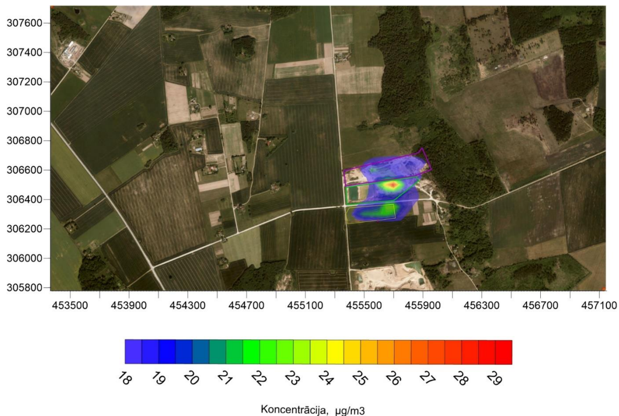
3.6.att. Daļiņu PM 10 gada vidējo koncentrāciju novērtējums. Esošā situācija.
