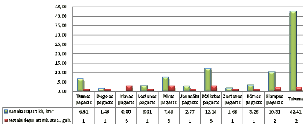
1.28.attēls. Tukuma novada kanalizācijas infrastruktūru raksturojošie rādītāji, 2011.g. sākums
