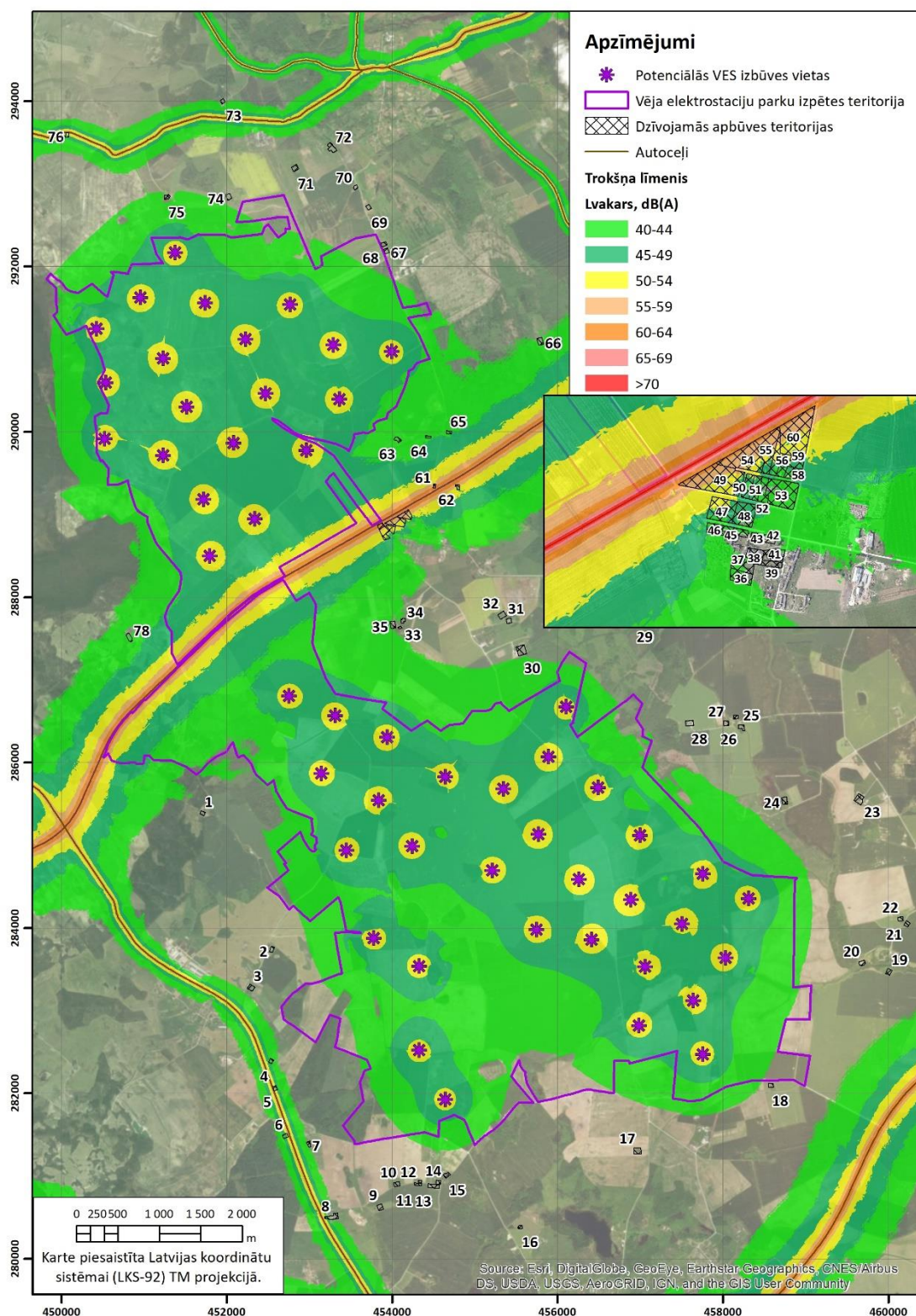
3.24. attēls. Aprēķinātais kopējais elektrostaciju radītais trokšņa līmenis vēja elektrostaciju parku izpētes teritorijas apkārtnē trokšņa radītājam L_{vakars} , vēja elektrostacijām darbojoties ar maksimālo skaņas jaudas līmeni (paredzēto darbību 2. alternatīva)
