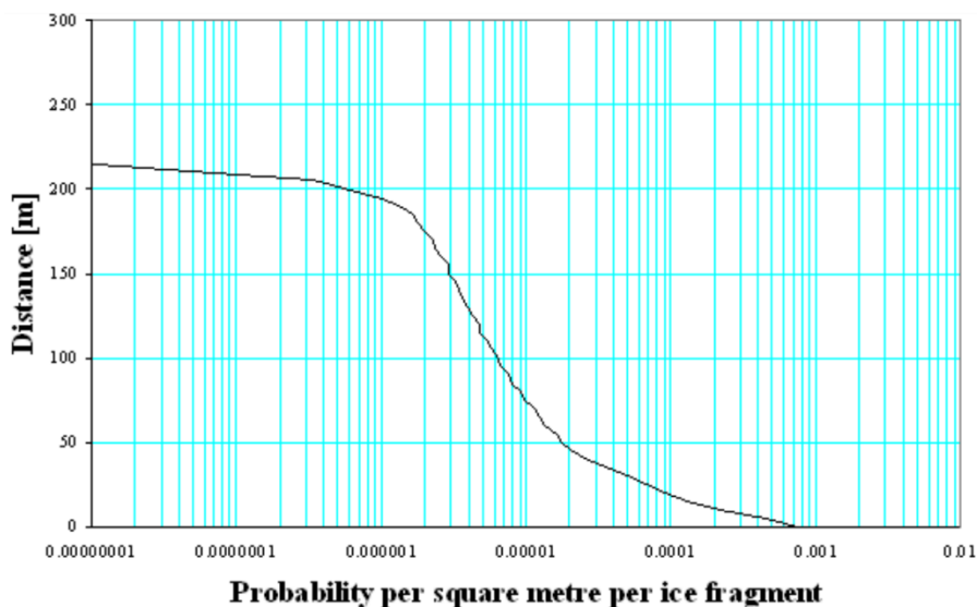
3.34. attēls. Ledus gabalu krišanas attāluma varbūtības aprēķini
