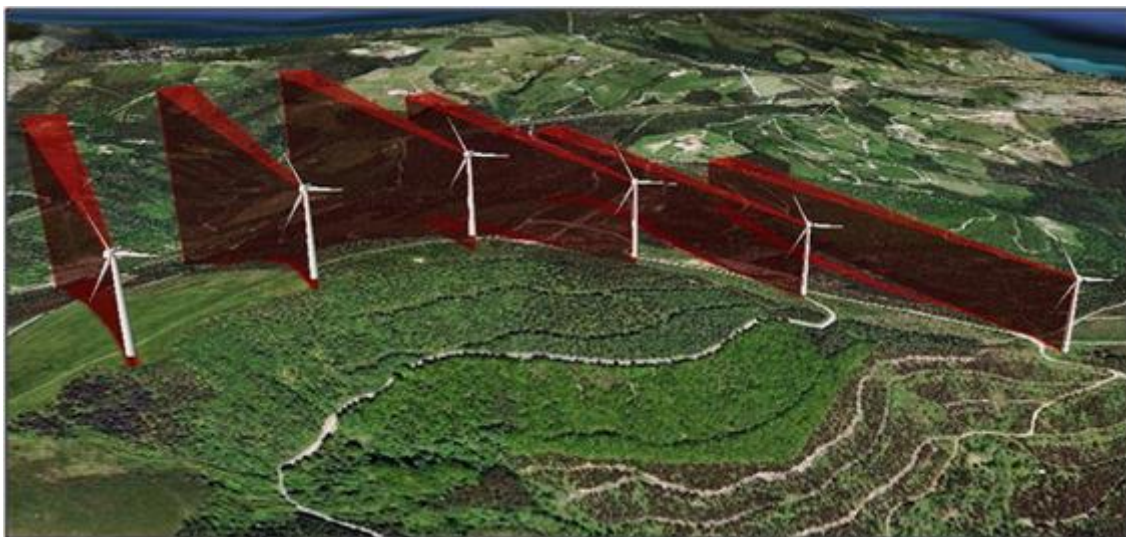
3.32. attēls. Aprēķinu piemērs par VES radītu zonu, kurā tiek bloķēts radara stars 42
