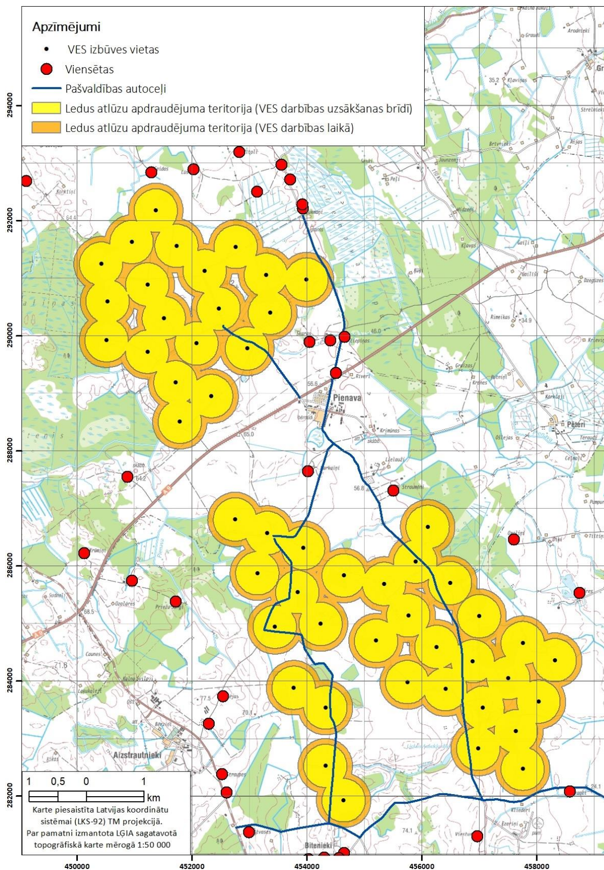
3.35. attēls. Iespējamā ledus atlūzu apdraudējuma zona
