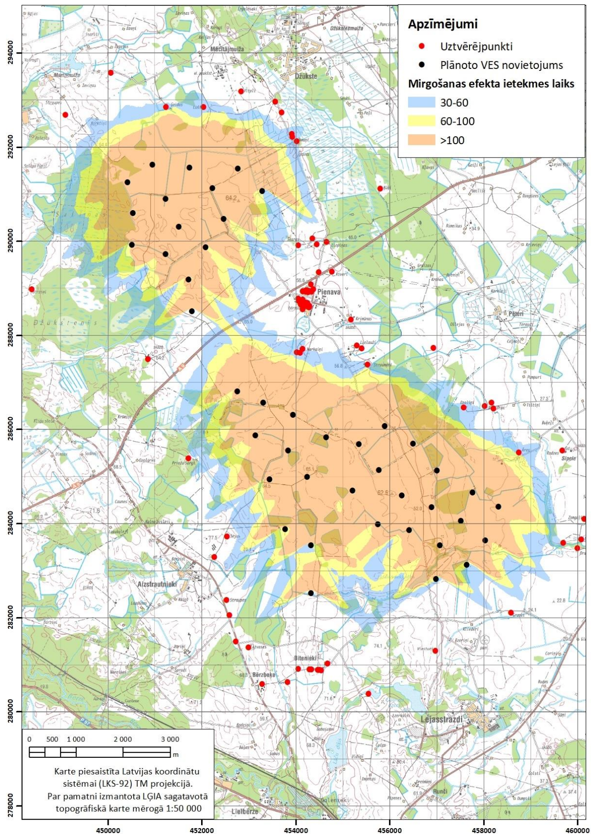
3.28. attēls. Mirgošanas efekta ietekmes laiks, kas aprēķināts pēc sliktākā scenārija metodes, plānoto ves parku 1. alternatīvām
