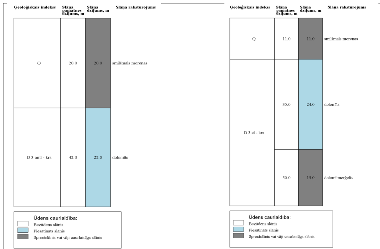
2.22. attēls. Īdensapgādes urbumu Nr. 10365 (pa kreisi) un 10364 (pa labi) ģeoloģiski tehniskie griezum (avots: LVĢMC uzturētā datu bāze "Urbumi")
