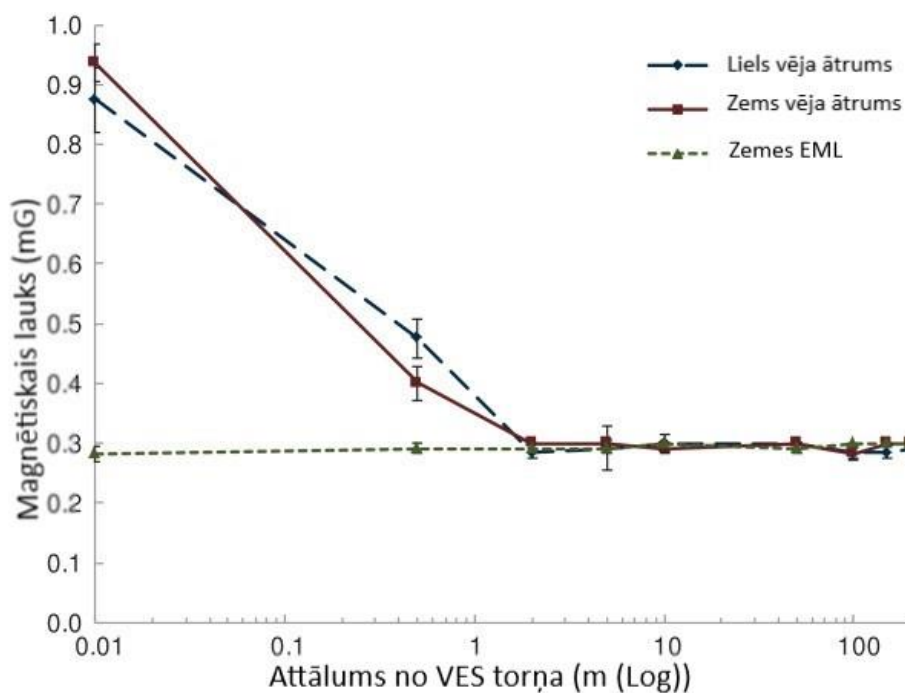
3.30. attēls. Elektromagnētiskā starojuma līmenis VES tuvumā 39
