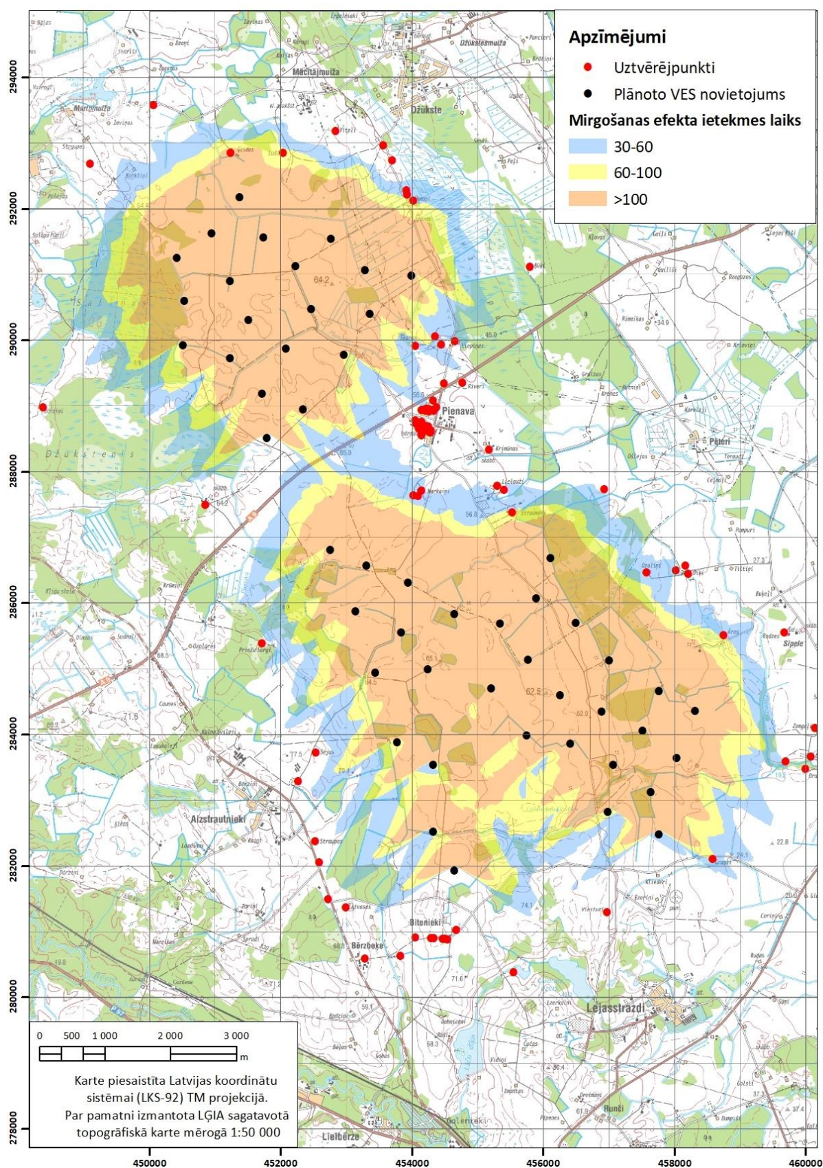
3.29. attēls. Mirgošanas efekta ietekmes laiks, kas aprēķināts pēc sliktākā scenārija metodes, plānoto ves parku 2. alternatīvām
